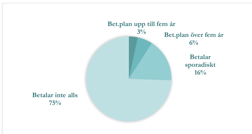
Diagram 1 Uppsagda lån
